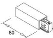
Einspeiser Schutzleiter rechts 600.118.1 schwarz 600.118.2 weiß 600.118.7 silber
